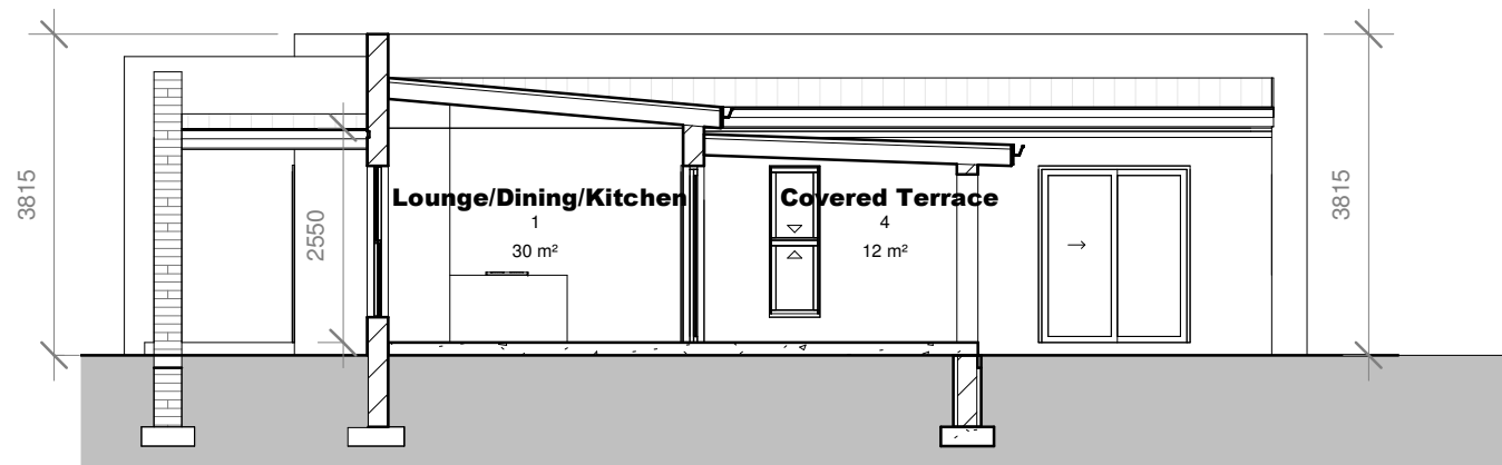
1 Section 1 1 : 100
